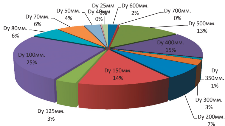
Рис.6. Распределение диаметров трубопроводов теплосети в процентном отношении от их протяжённости.
