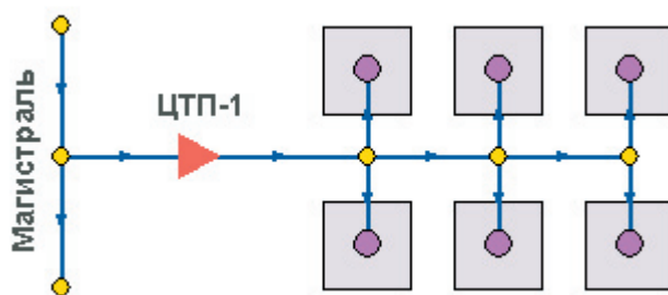
Рис. 3.4. ЦТП
