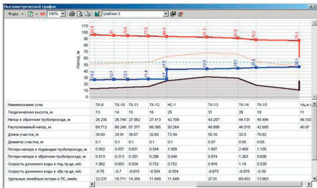
Рис. 3.13. Пьезометрический график
