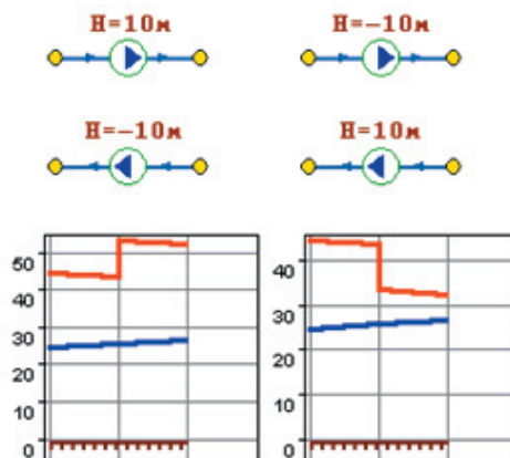
Рис. 3.8. Пьезометрические графики
