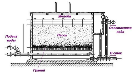
Контактный осветлитель
